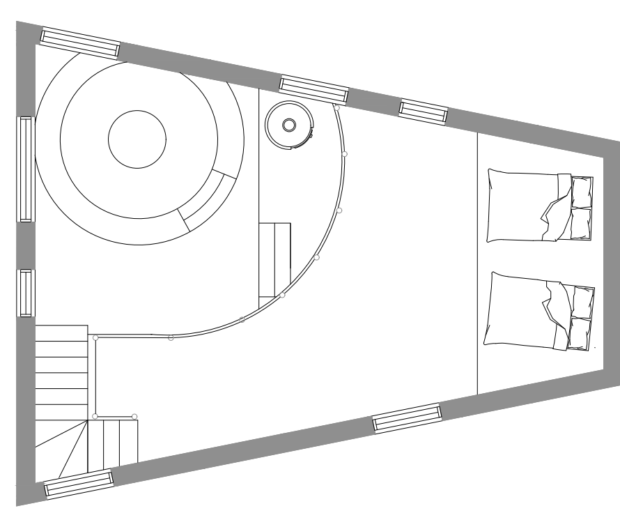
Plan habitation à 2 niveaux // Mezzanine 1:100
