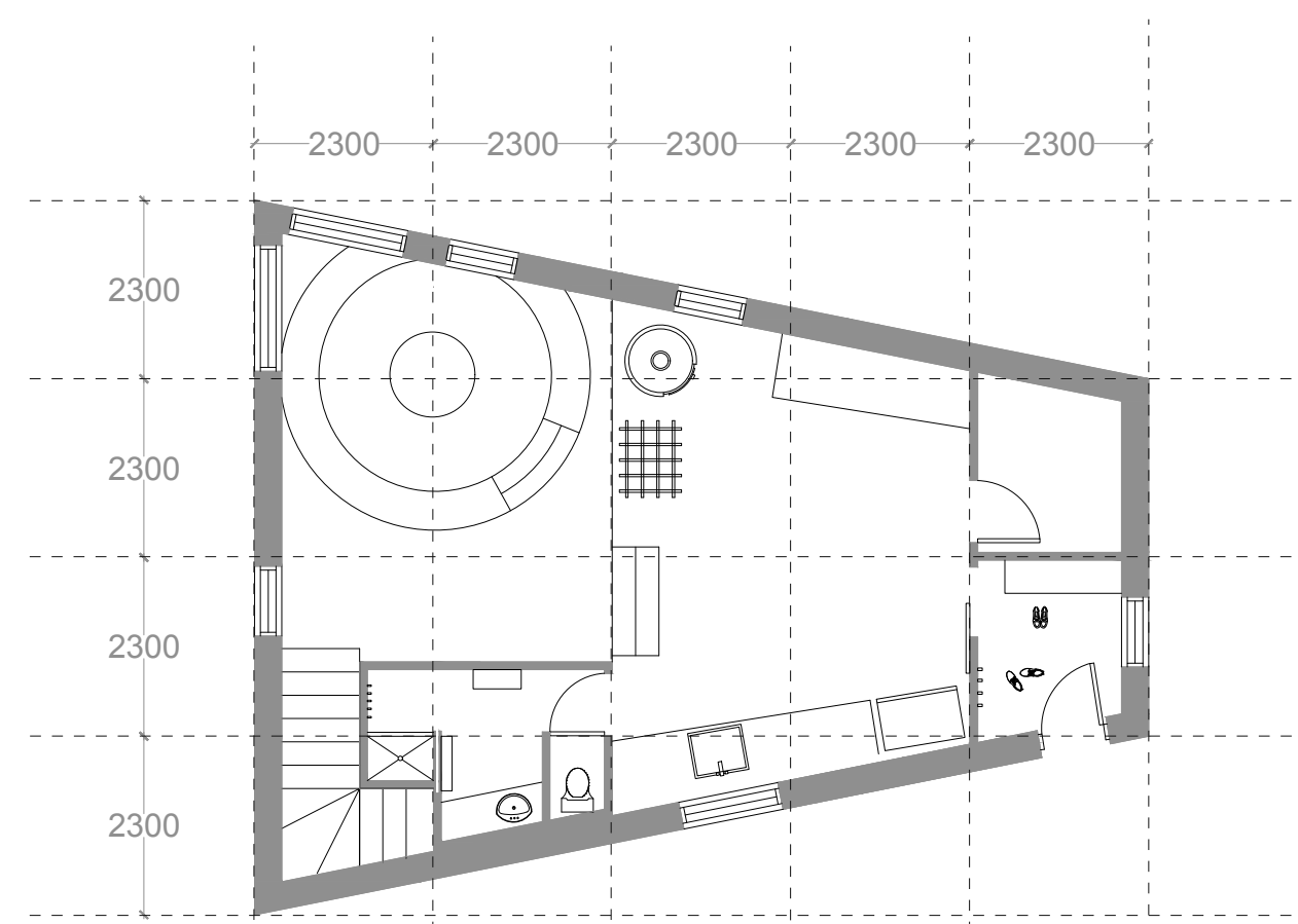
Plan habitation à 2 niveaux // RDC 1:100
