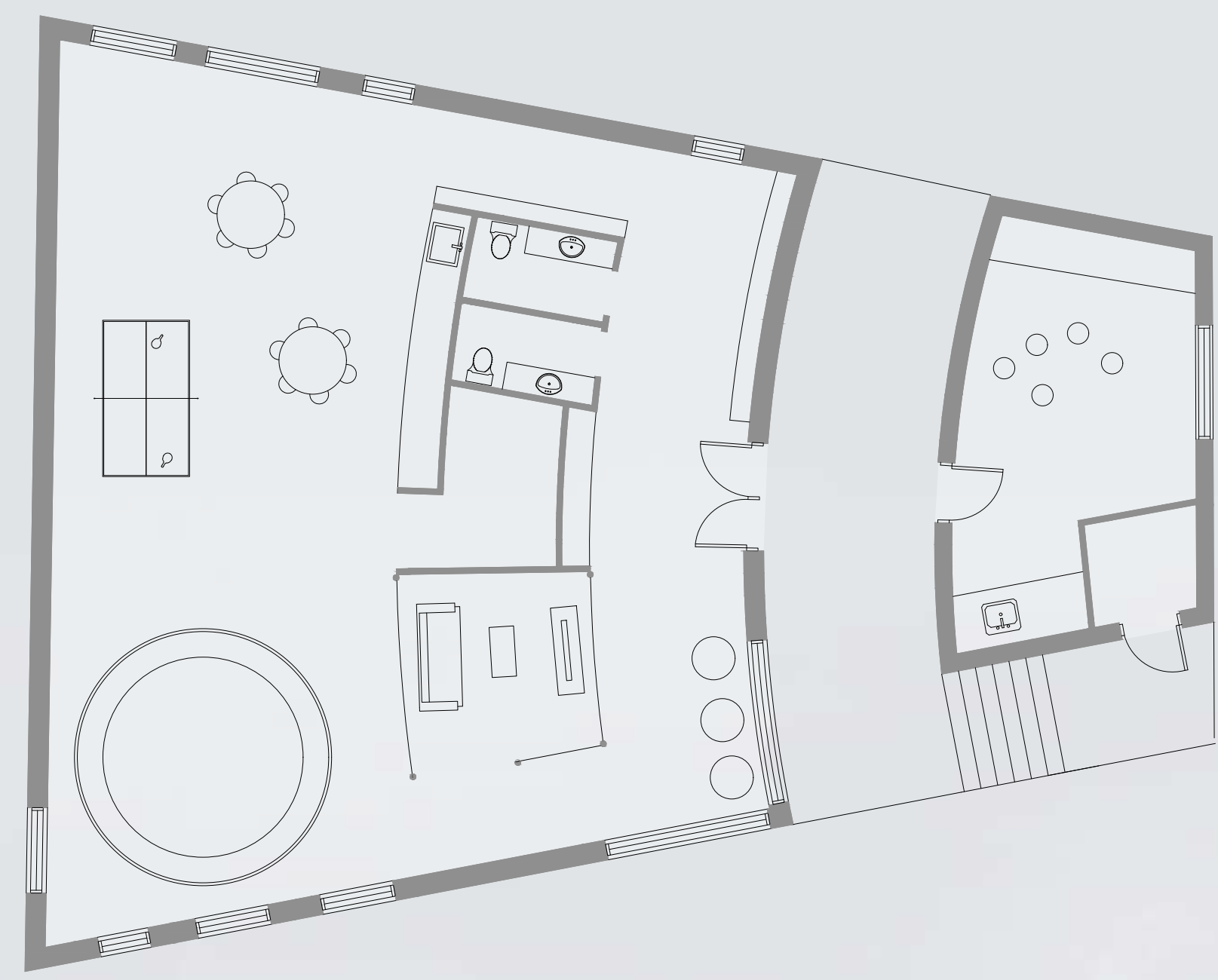
Plan centre communautaire 1:100
