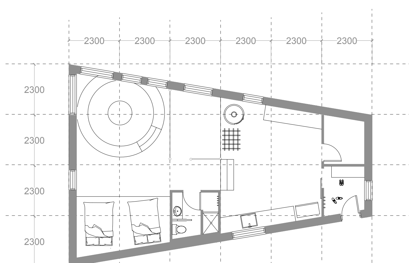
Plan habitation à 1 niveau 1:100
