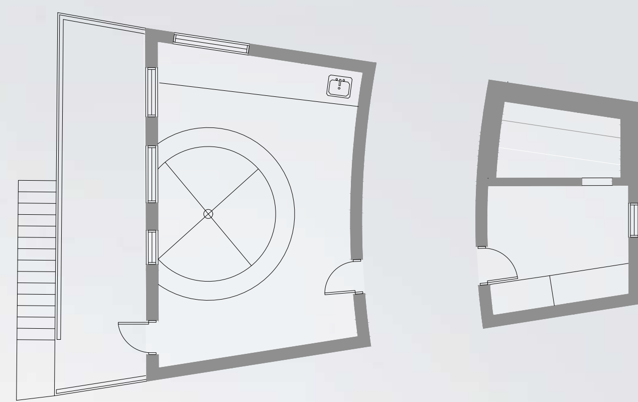
Plan atelier de chasse et pêche 1:100
