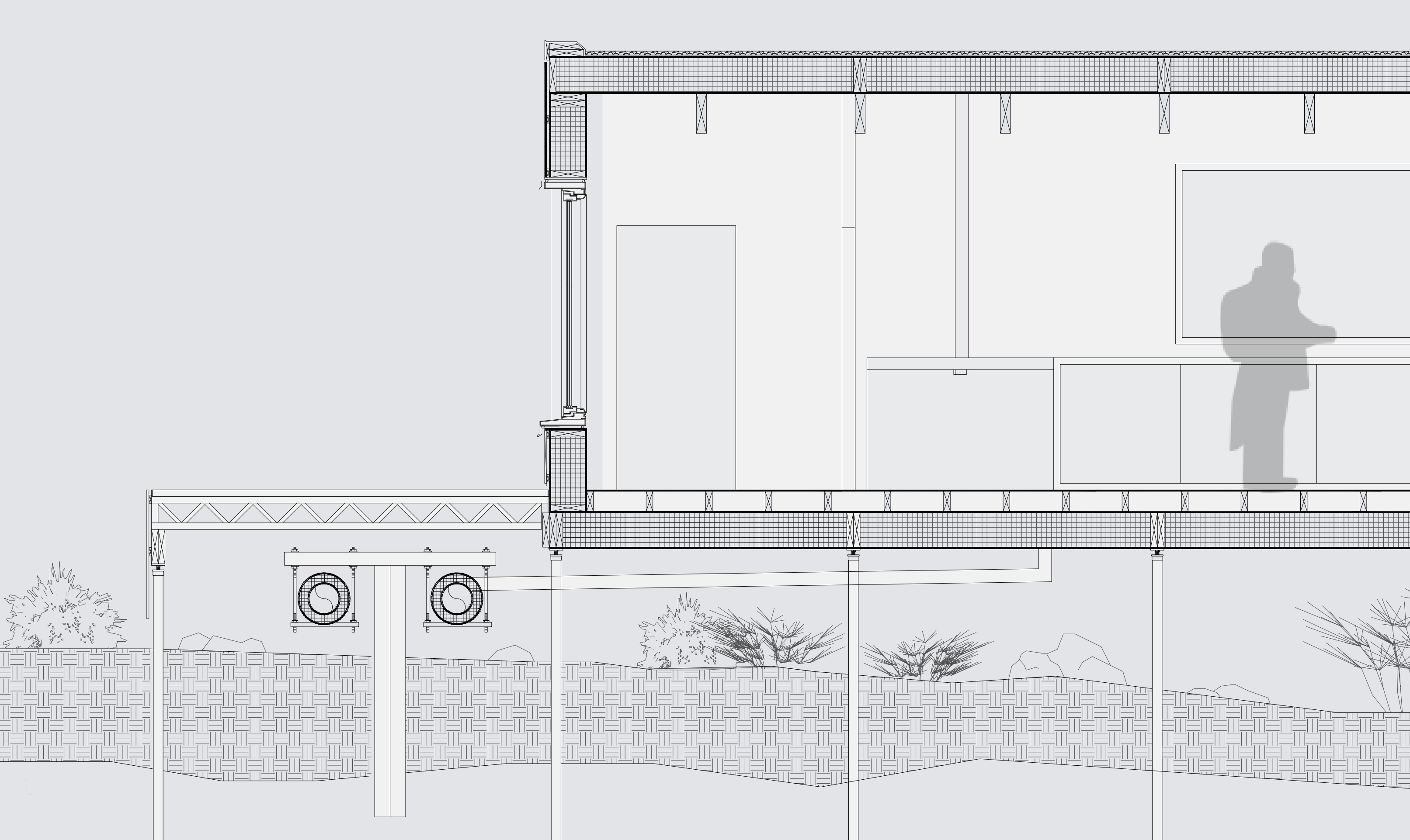
Détail constructif 1:25
